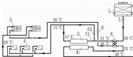
1. 间接蒸发冷水机组; 2. 机械制冷冷水机组蒸发器; 3. 机械制冷冷水机组冷凝器; 4. 显热末端; 5. 新风机组冷却盘管; 6、7. 冷水循环泵; 8. 换热器; F1、F2. 转换阀门。
